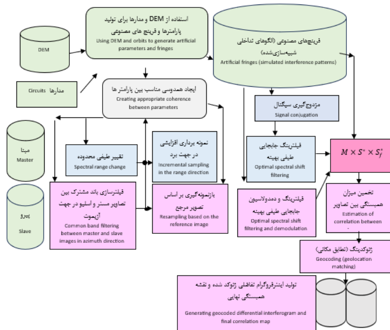
شکل ۱: فلوچارت مراحل طی شده در پردازش تصاویر راداری Fig. 1: Flowchart of the steps taken in processing radar images
