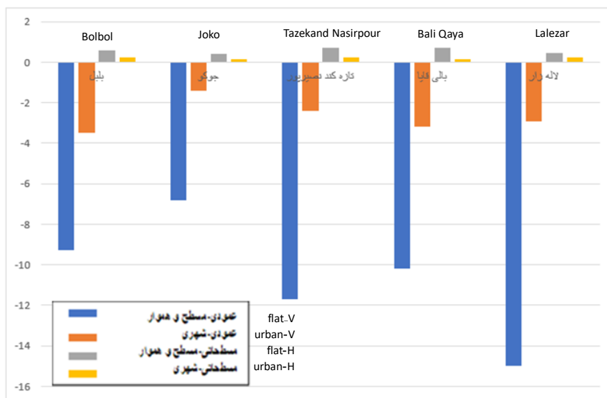
شکل ۱۱: نمودار مقایسه‌ی تغییرات سطح زمین با تصاویر اپتیک و تکنیک تبدیل (فتوگرامتری پهپادی) برحسب سانتی‌متر Fig. 11: Chart comparing changes in land surface with optical images and conversion techniques (UAV photogrammetry) in centimeters
