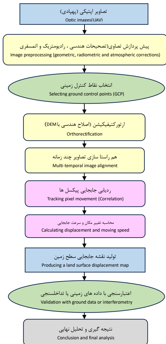
شکل ۶: فلوچارت مراحل طی شده در پردازش تصاویر اپتیک Fig. 6: Flowchart of the steps taken in optical image processing
