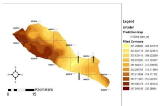
شکل ۱۶: نقشه پیش‌بینی حاصل از درون‌یابی به روش کریجینگ معمولی بر اساس مدل دایره‌ای Fig. 16: Prediction map resulting from interpolation using the normal kriging method based on the circular model
