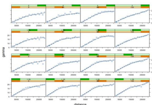
شکل ۷: بررسی همسانگردی داده‌ها در جهت‌های مختلف Fig. 7: Examining data isotropy in different directions
